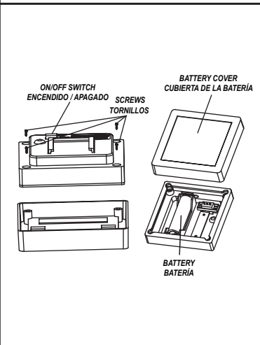
SOME PARTS MAY COME PRE-ASSEMBLED ALGUNAS PARTES QUIZÁ YA PUDIERAN ESTAR ENSAMBLADAS
